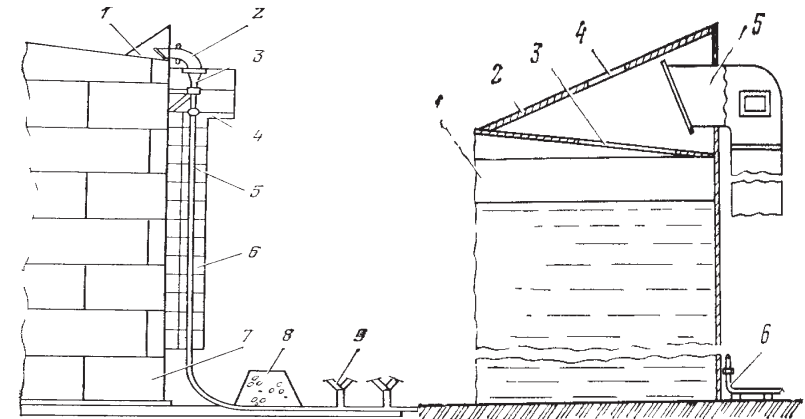
Рис.15.4. Схема стаціонарної установки генератора піни на резервуарі: 1 – пристосування з легкоплавкими замками, що герметизує пінокамеру; 2 – пінокамера; 3 – піногенератор; 4 – площадка обслуговування генератора піни, 5 – трубо-провід для подачі розчину піноутворювача; 6 – драбина для підйому на площадку; 7 – резервуар; 8 – обвалування; 9 – розгалуження трубопроводів для підключення рукавів пожежного автомобіля
