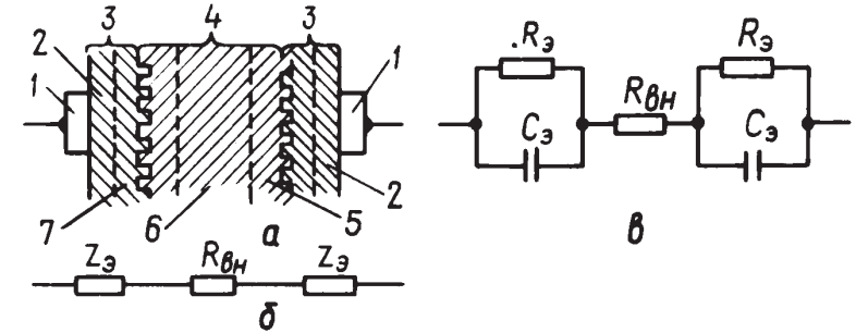
Рис.12.1 Схема електричного опору у тіла людини: a – схематичне зображення ввімкнення тіла людини в електричний ланцюг; б, в – еквівалентні схеми електричного опору тіла людини; 1 – електроди; 2 – роговий шар шкіри; 3 – зовнішній шар шкіри – епідерміс (роговий і паростковий шари); 4 – внутрішні шари шкіри і підшкірні тканини; 5 – внутрішній шар шкіри – дерма; 6 – підшкірні тканини; 7 – паростковий шар шкіри; Z_e – повний електричний опір епідермісу; R_{вн} – опір внутрішніх тканин; R_e – активний опір епідермісу; C_e – ємність конденсатора
