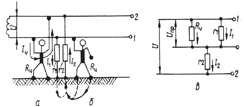
Рис.12.2. Схеми дотику до двопровідної мережі: а – двополосний дотик; б – однополосний дотик; в – схема заміщення (випадок однополосного дотику)
