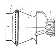
Рис. 15.3. Генератор піни середньої кратності (ГПС)
