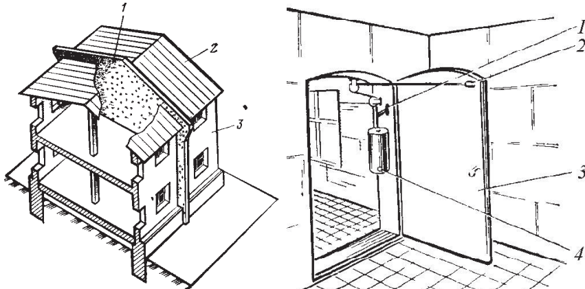
Рис. 14.2. Протипожежна стіна: 1 – протипожежна стіна; 2 – металева покрівля; 3 – стіна, що згорає.
