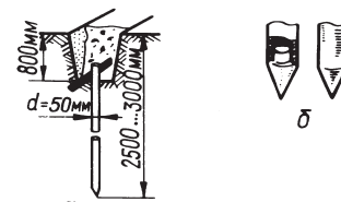
Рис.12.7. Установка одиночного стержневого заземлителя в траншее: а – общий вид; б – наконечники стержневых заземлителей
