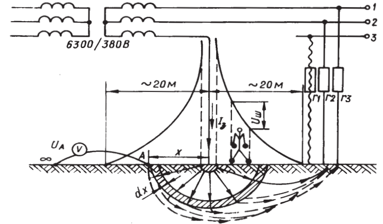
Рис.12.3. Розподіл потенціалу по поверхні землі навколо напівкульового заземлювача
