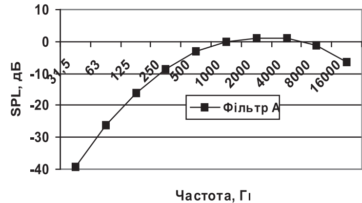
Рис.8.2. Шкала коригування вимірювача А на різних частотах
