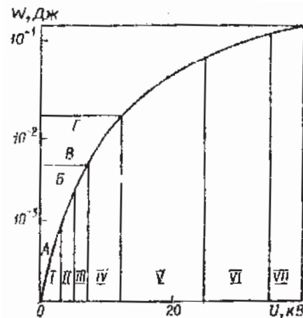
Рис.13.2. Оцінка небезпеки електростатичних розрядів на людину
