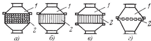
Рис. 14.1. Вогнезагороджувачі: а – насадочний; б – пластинчастий; в – касетний; з – сітчастий; 1 – корпус; 2 – насадка (кульки скляні, гравій, касета з пластин, сітки)
