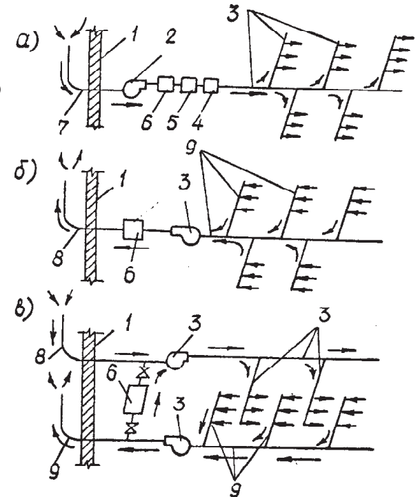
Рис. 3.2. Схема видів штучної (механічної) вентиляції:
