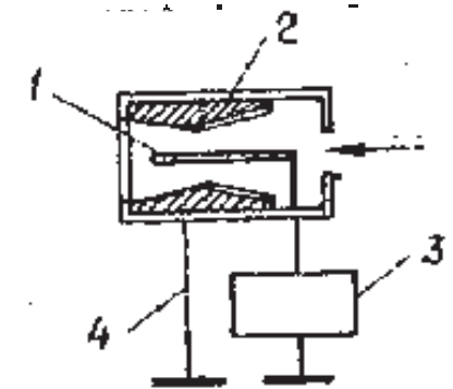
Рис.13.6. ІЕГД нейтралізатора: 1 – високовольтний електрод; 2 – надзвукове сопло; 3 – ДВН; 4 – мережа заземлення
