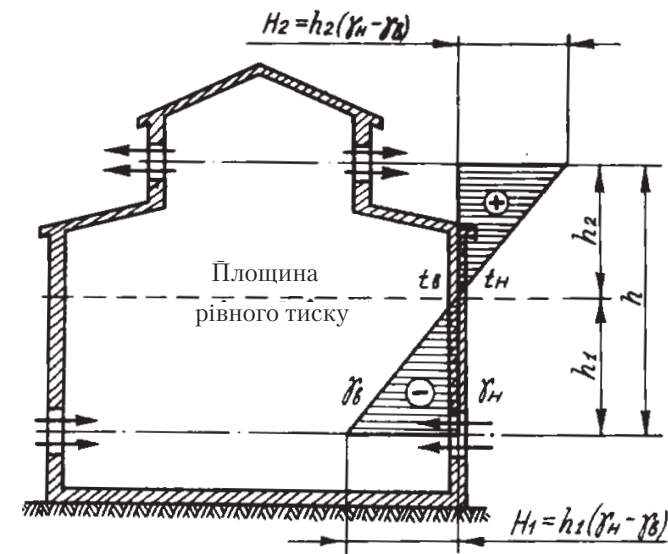
Рис. 3.1. Принцип роботи природної вентиляції
