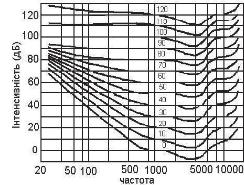
Рис.8.1. Криві однакової гучності
