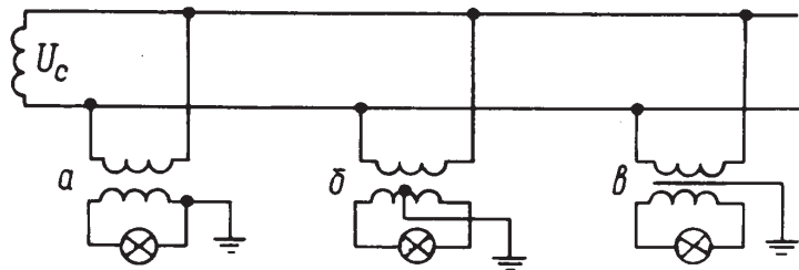
Рис.12.5. Схема захисту людини при переході напруги з високовольтної обмотки в обмотку малої напруги в мережах з напругою до 1000 В: а – заземлення одного з кінців обмотки малої напруги; б – заземлення середньої точки; в – заземлення екранувальної обмотки (екрана).
