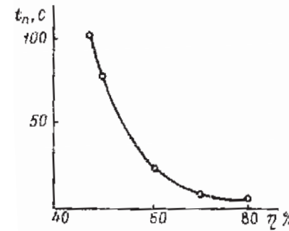
Рис.13.3.Підвищення антистатичних властивостей матеріалів з ростом відносної вологості
