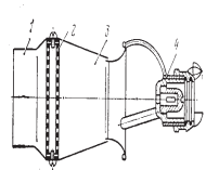
Рис. 15.3. Генератор піни середньої кратності (ГПС)
