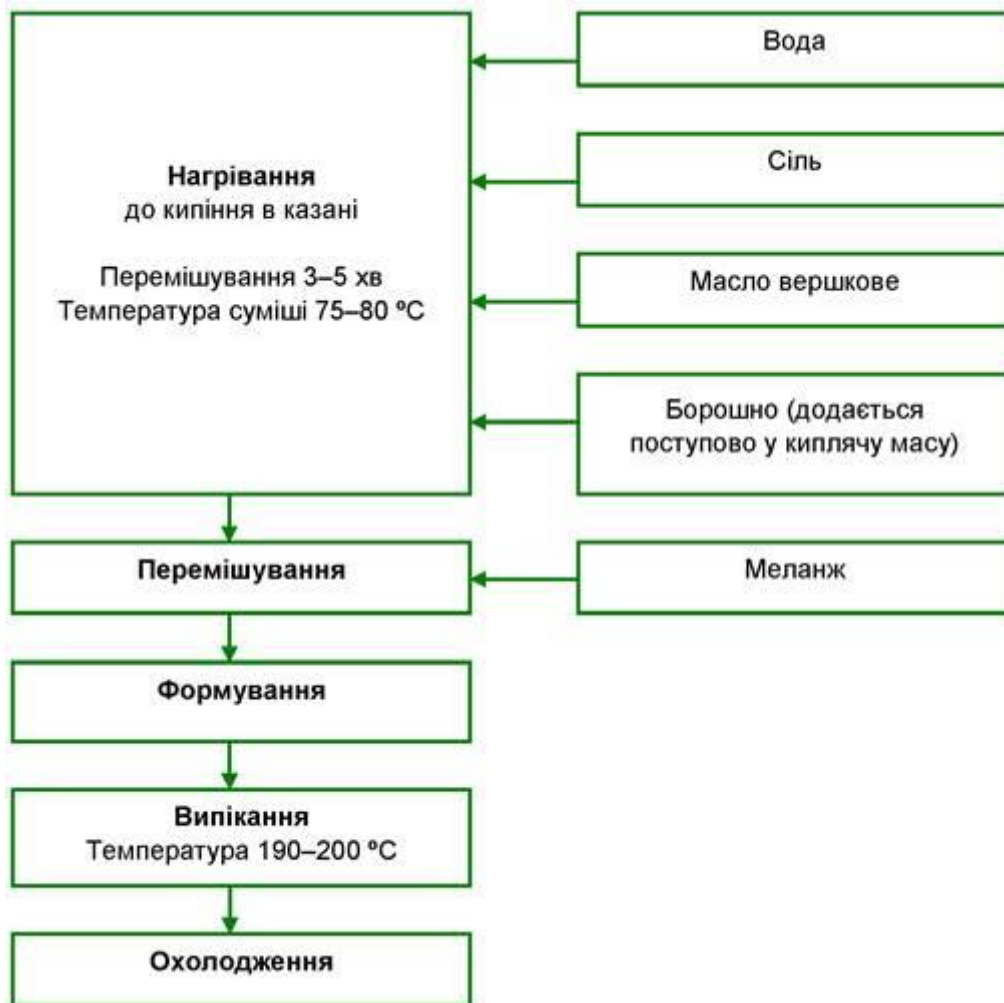
Технологічна схема приготування заварного напівфабрикату
